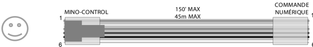
Figure 20 – Configuration du branchement pour une seule commande numérique murale. Cette configuration depuis le no de série 21Q30601, utilisez celle du visage triste sinon.
