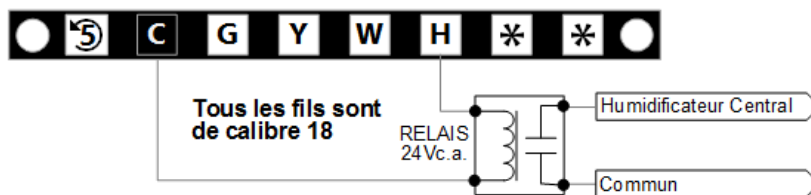
Figure 17 - Branchement à un humidificateur à contacts nets requérant l’usage d’un relais.
