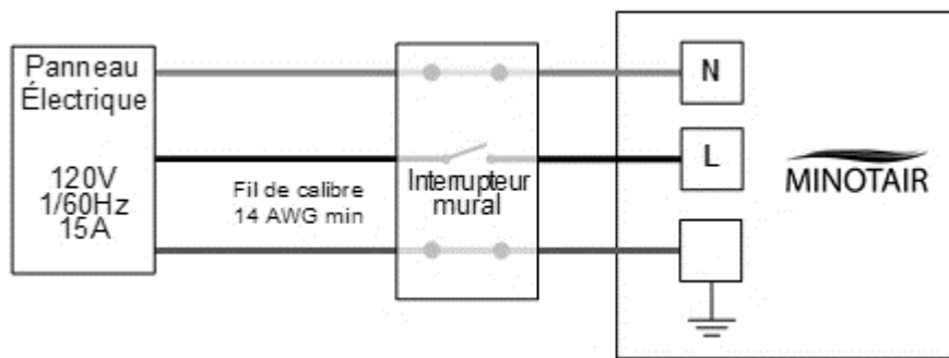
Figure 25 – Branchement de l'appareil.
