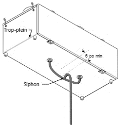
Figure 15 – Positionnez l'adaptateur en Té de façon à former un siphon.
